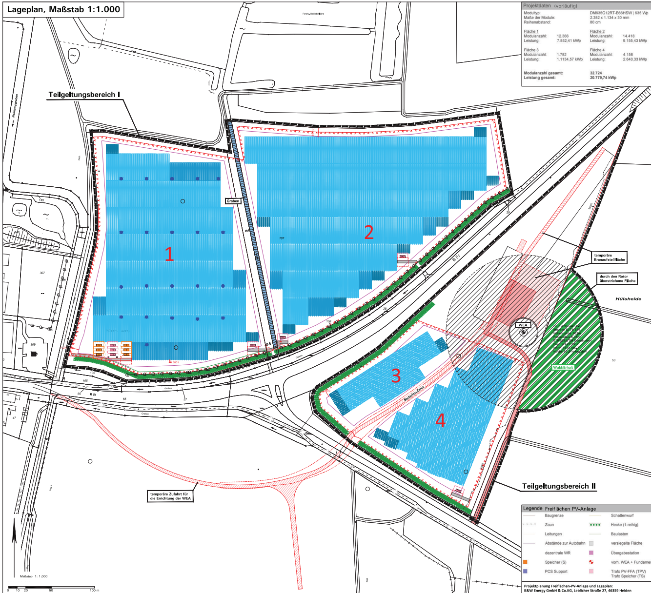
Lageplan, Maßstab 1:1.000
