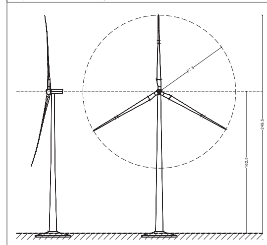
Windenergieanlage, Maßstab 1:1.000 (beispielhaft vermaßte Schnittzeichnungen)
