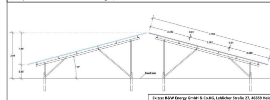
Schnitt PV-Anlage, ohne Maßstab (beispielhaft vermaßte Schnittzeichnungen)
