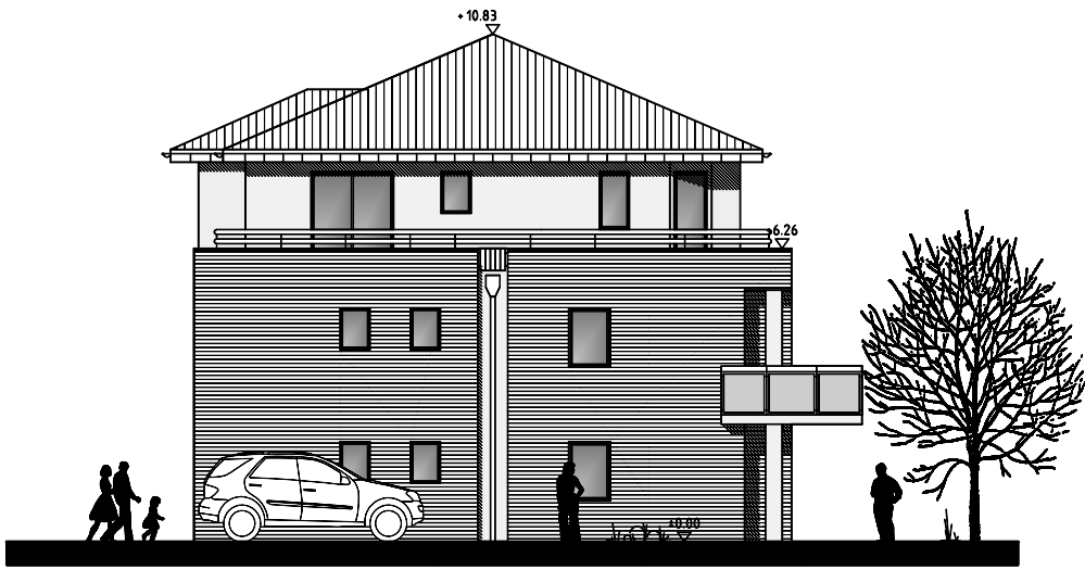
Ansicht Westen Haus 1
