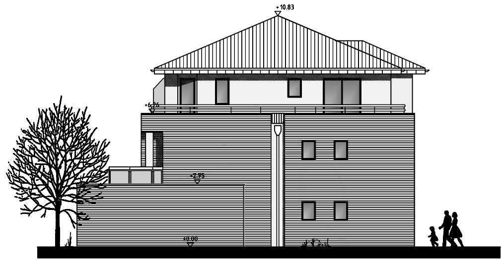
Ansicht Osten Haus 1
