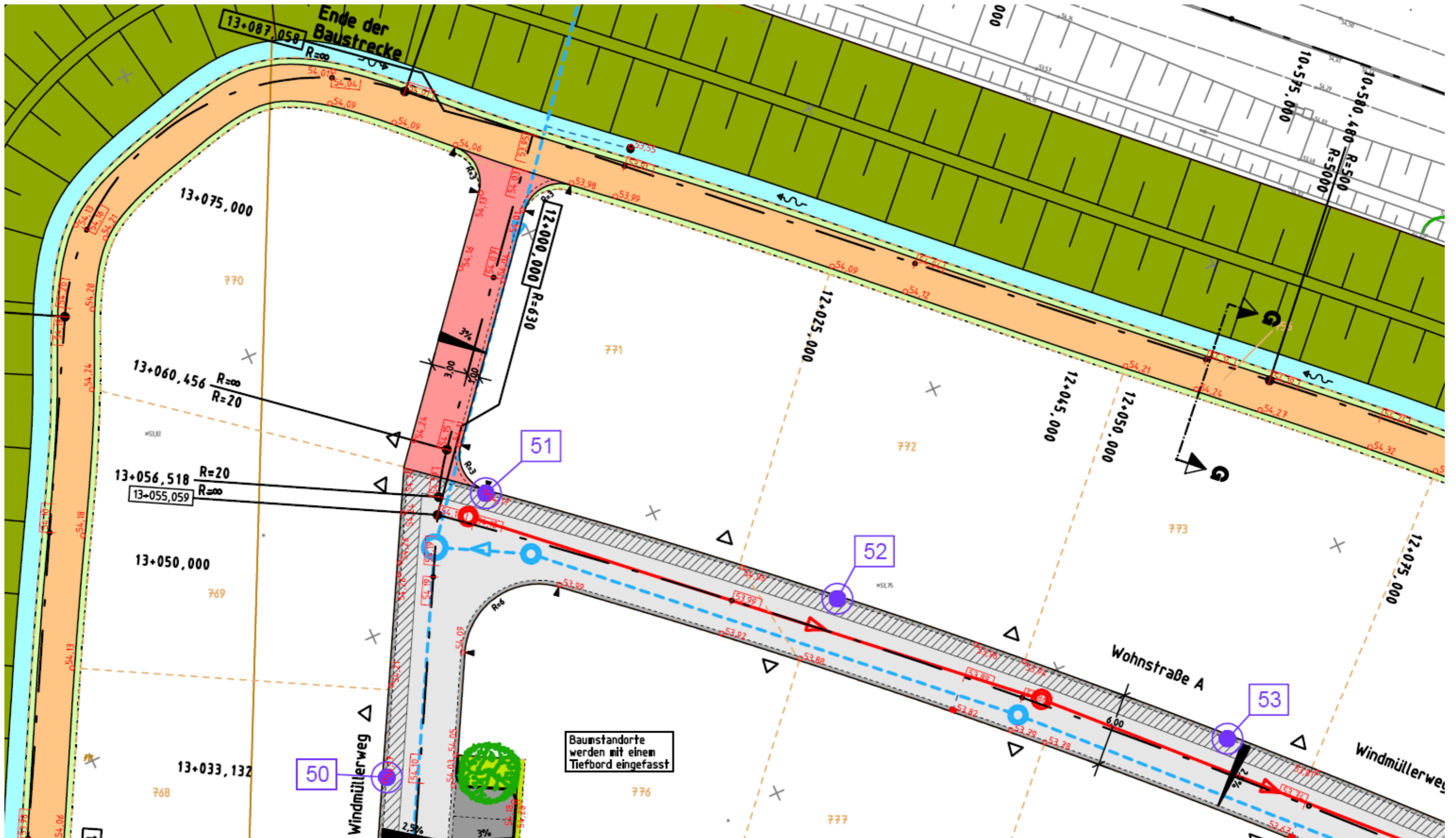
Auszug aus der Straßenplanung
