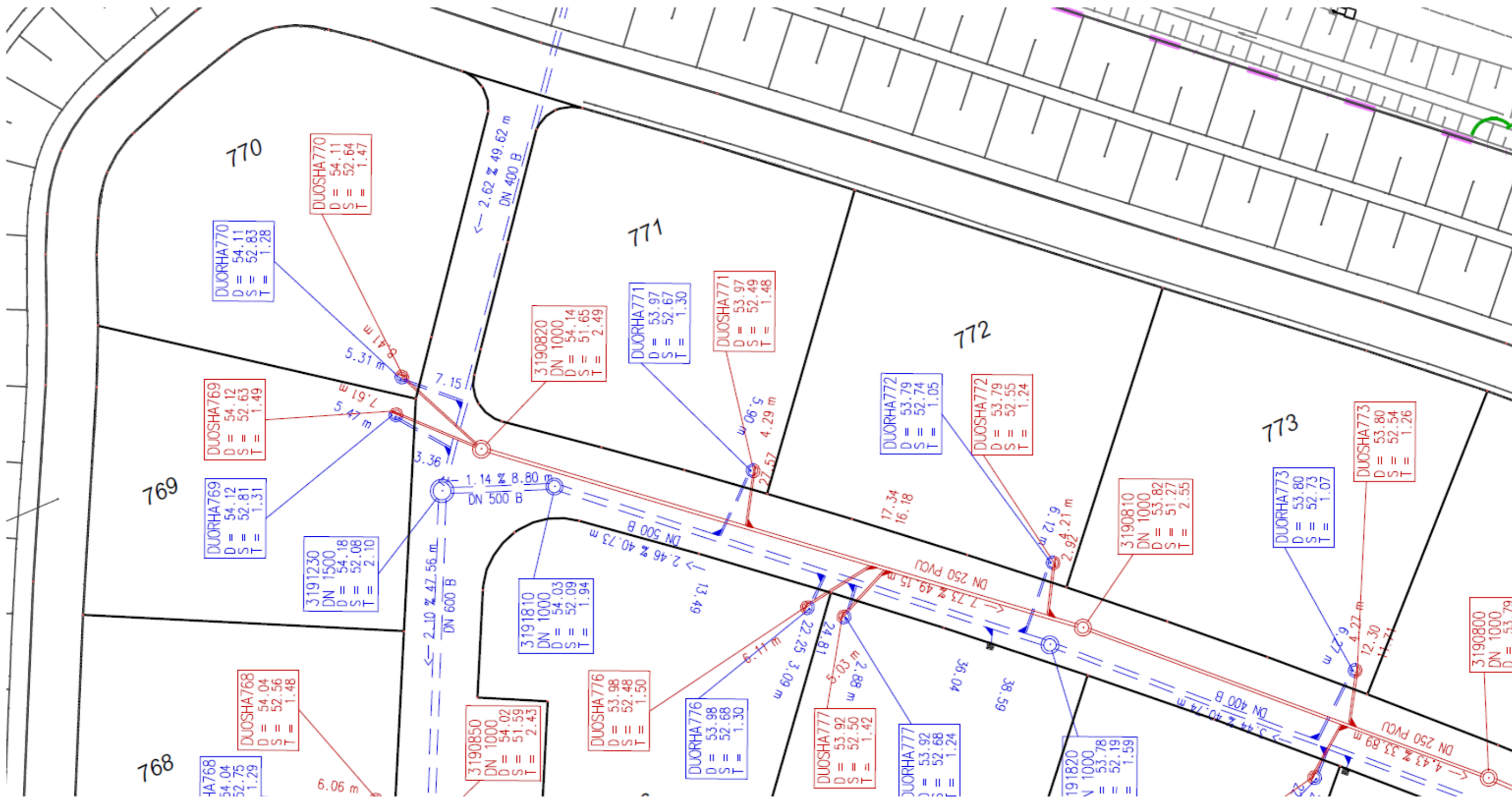
Auszug aus dem Kanalbestandsplan
