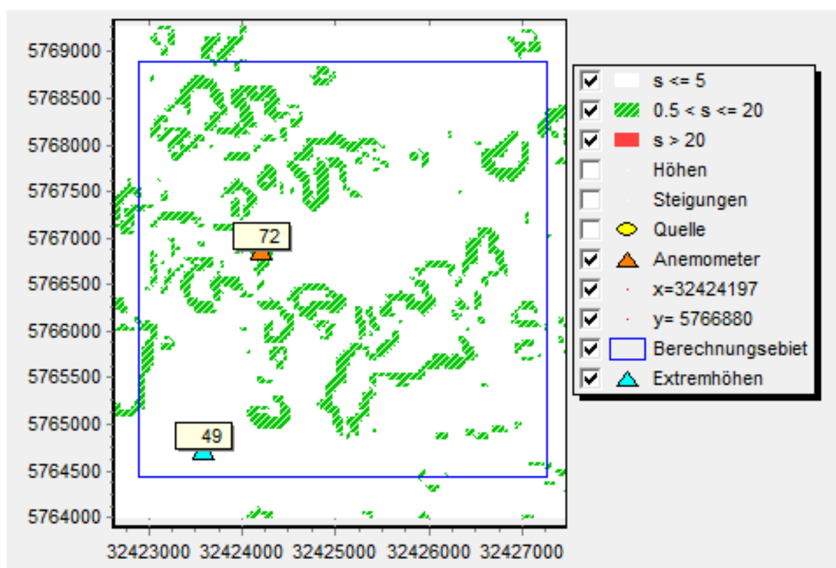
Abbildung 2 Steilheit und Anemometerposition im Rechenggebiet
